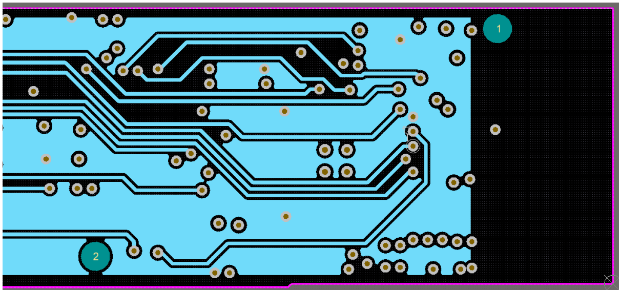
Layer 2
