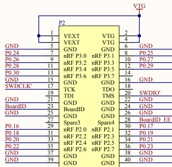
Samtec SFC-120-T2-L-D-MOD B
