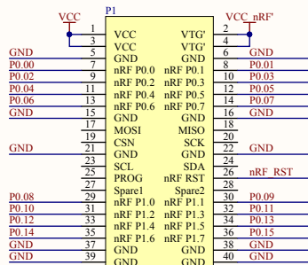
Samtec SFC-120-T2-L-D-MOD A
