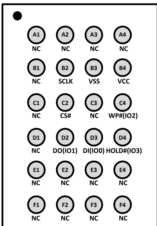
24-ball TFBGA
