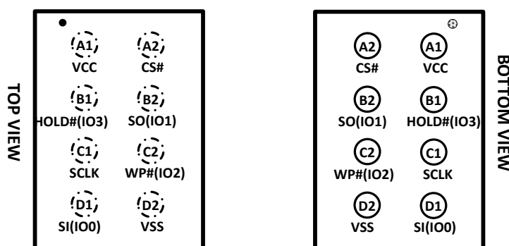
8-ball WLCSP
