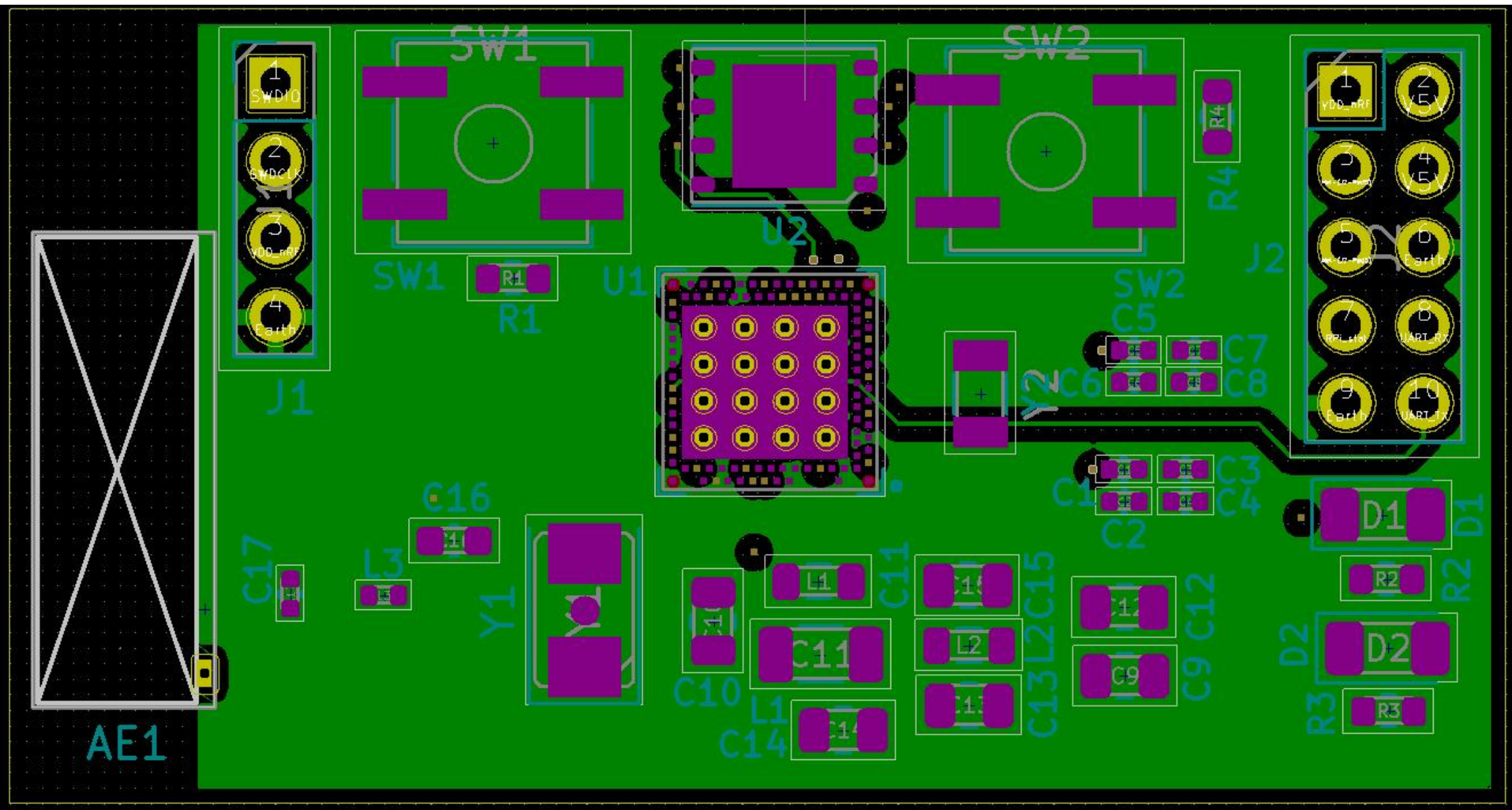
Bottom layer
