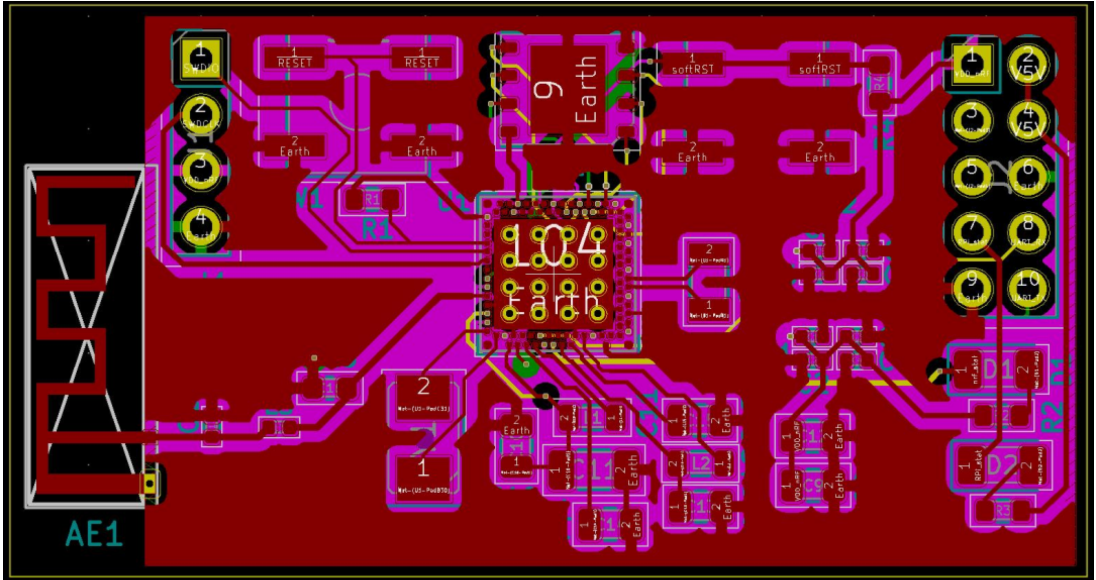
Front Layer
