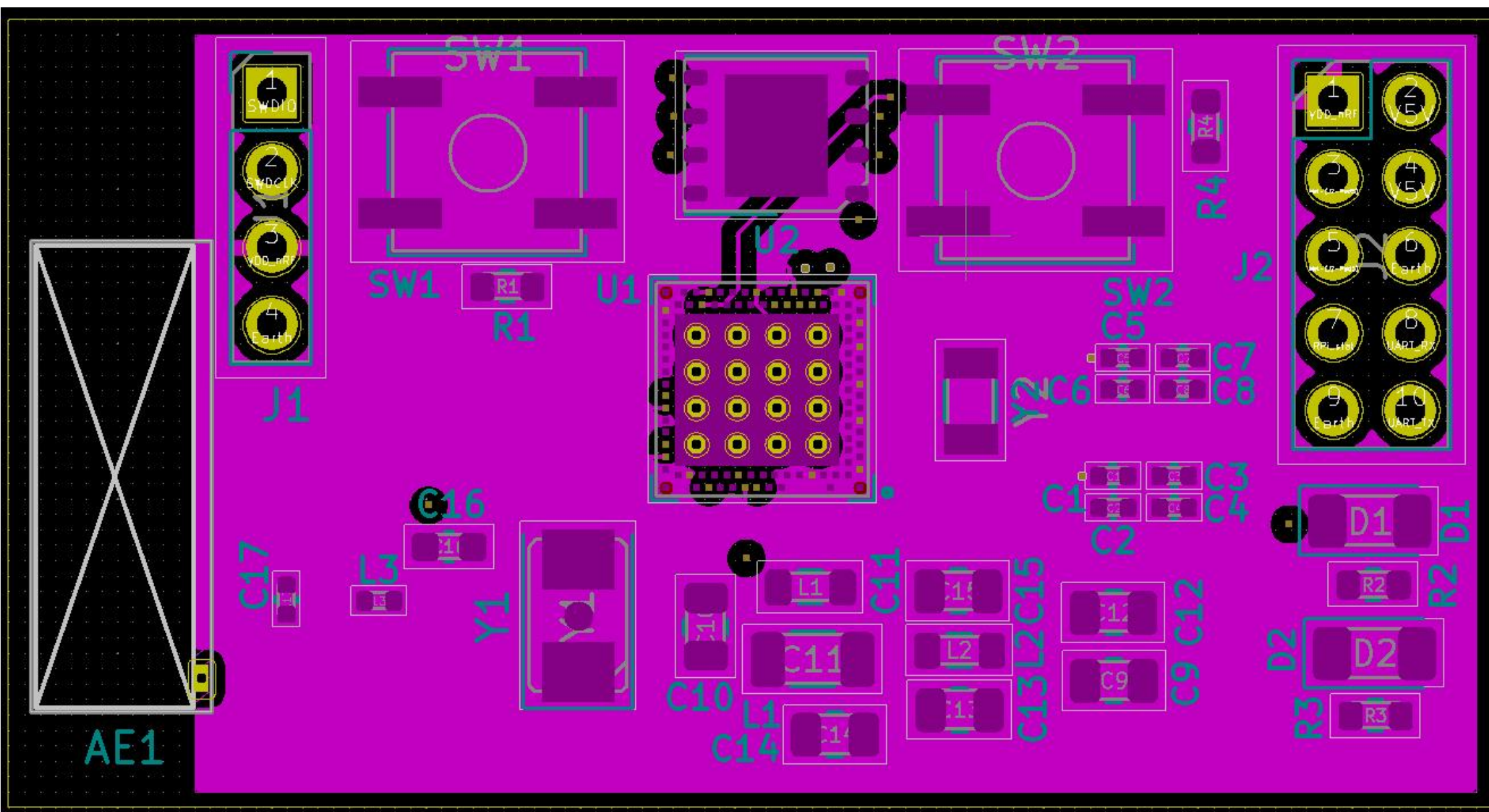
Inner Layer 2
